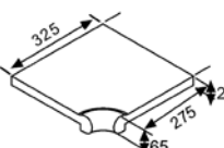
Remate esquina interior Internal edge
